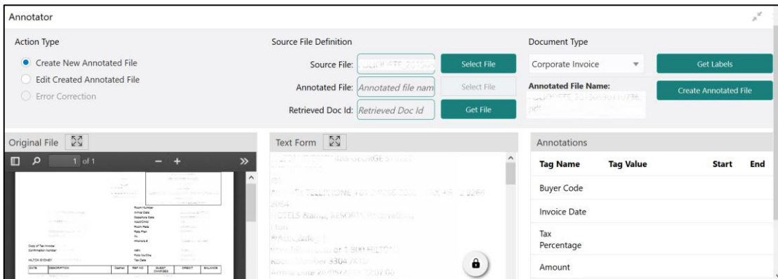
Figure 240: Tags
